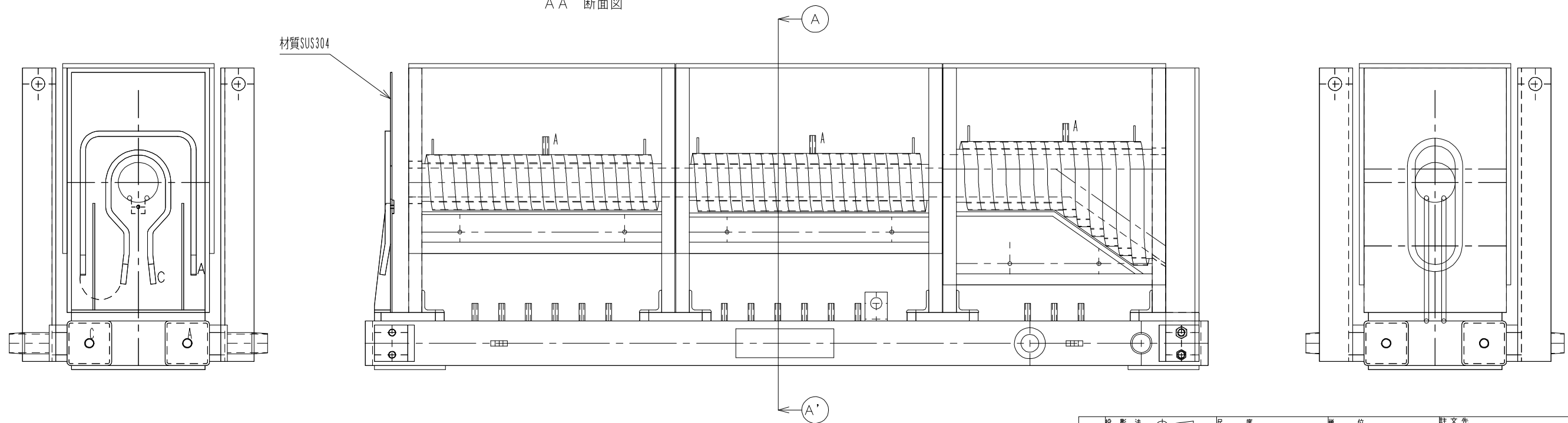
1/5断面図
